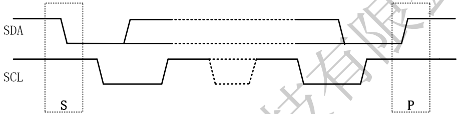
图 11-1 I 2 C 起始条件及终止条件
