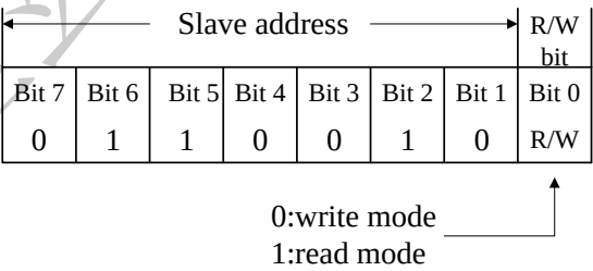
图 11-2 I 2 C 从地址示意
