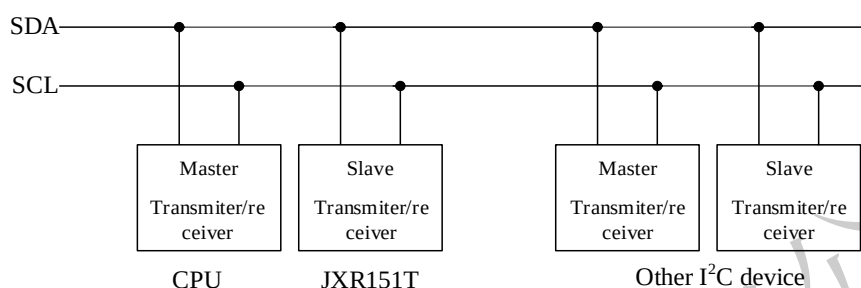
图 11-3 I 2 C 系统配置
