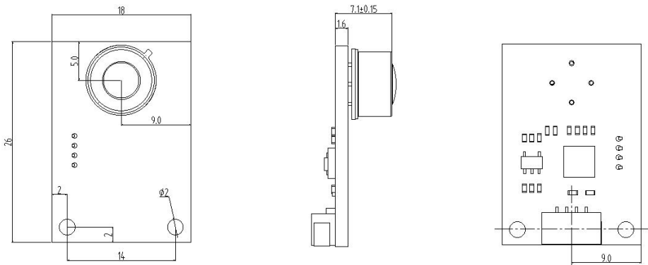
单位：mm 未标注尺寸公差：±0.1mm
