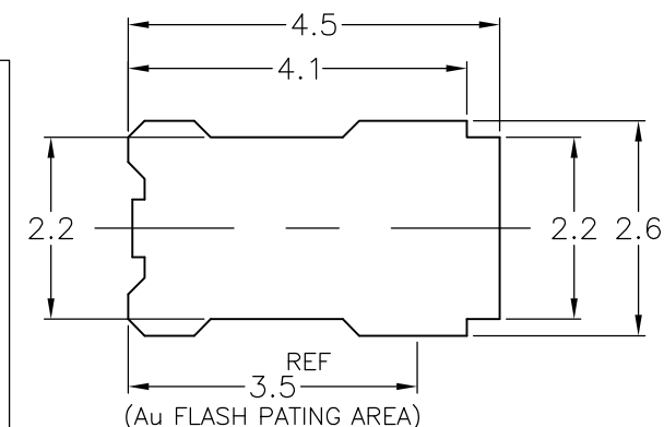
参考パッド寸法 RECOMMENDED FOOT PRINT REFERENCE ONLY
