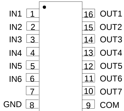
SO-16/TSSOP-16
