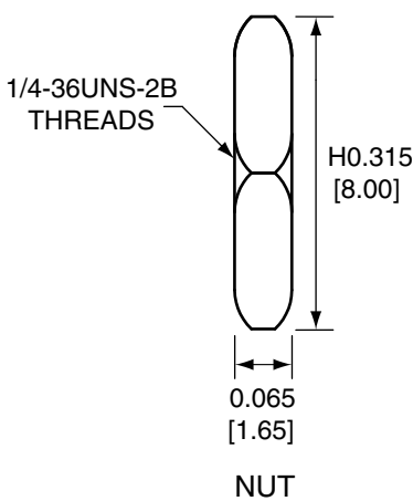
NUT
