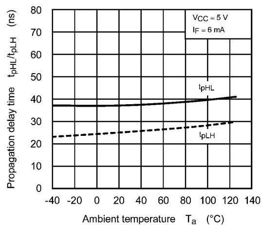
Fig. 12.2.11 t_{pHL}/t_{pLH} - T_a
