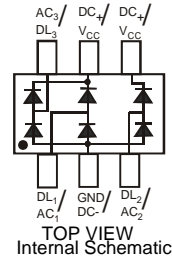
SOT-363
