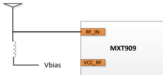
图 9-2 MXT909 其他电压范围的有源天线方案
