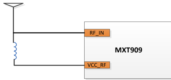
图 9-1 MXT909 3.3V 有源天线方案
