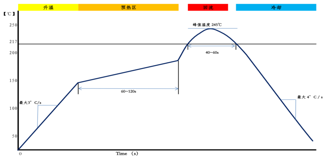
图 9-7 MXT909 推荐炉温曲线
