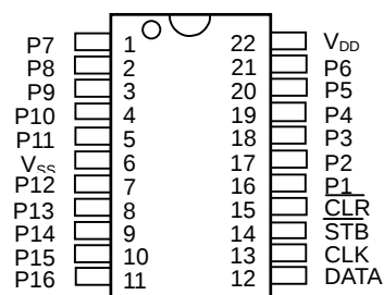
NJU3715L
