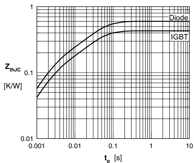
Fig. 14 Typ. transient thermal impedance
