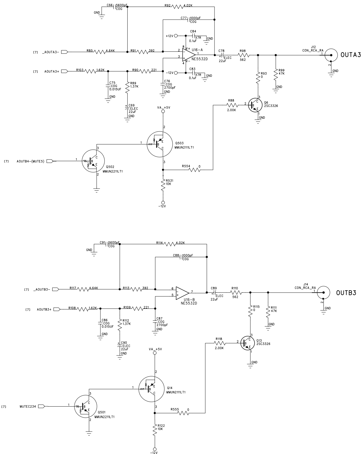
Figure 47. Analog Outputs A3 - B3
