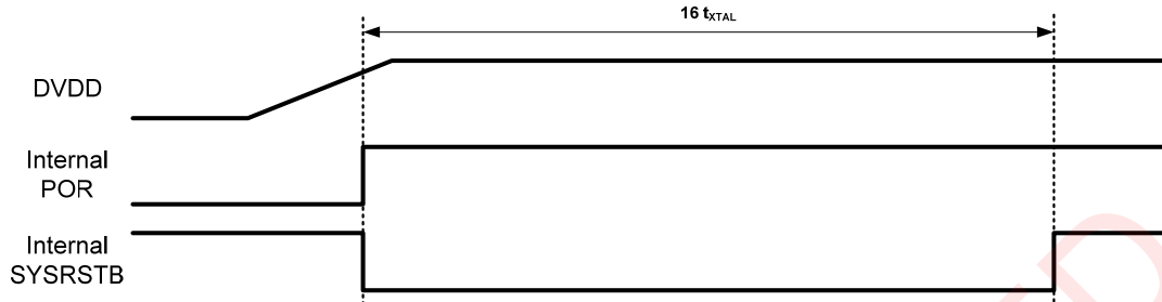
Figure 34 – POR Timing
