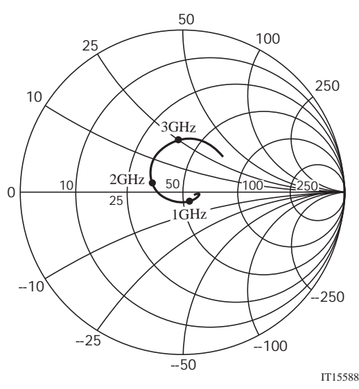
S Parameter S11
