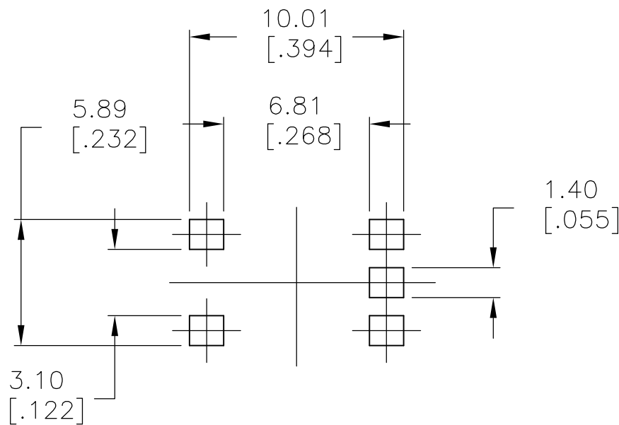
P.C.B. FOOTPRINT
