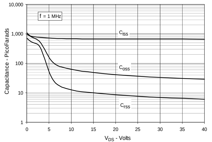
Fig. 10. Capacitance
