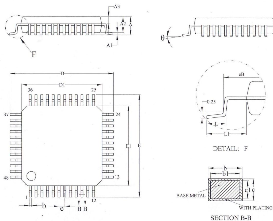
图 24 LQFP48-7x7mm, 48 脚低剖面方形扁平封装图
