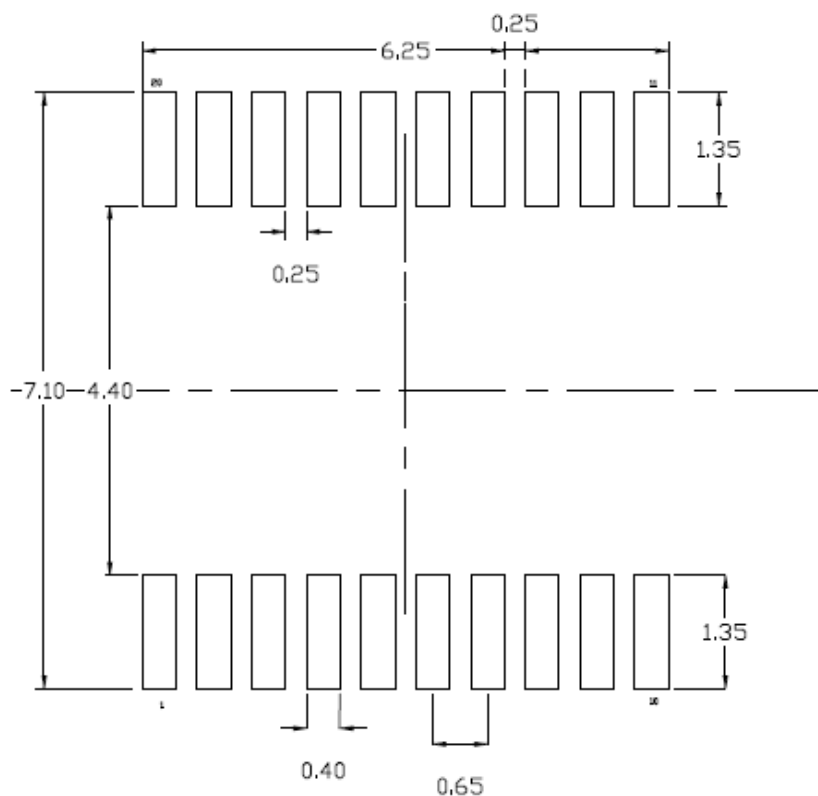
图 29 TSSOP20 推荐封装
