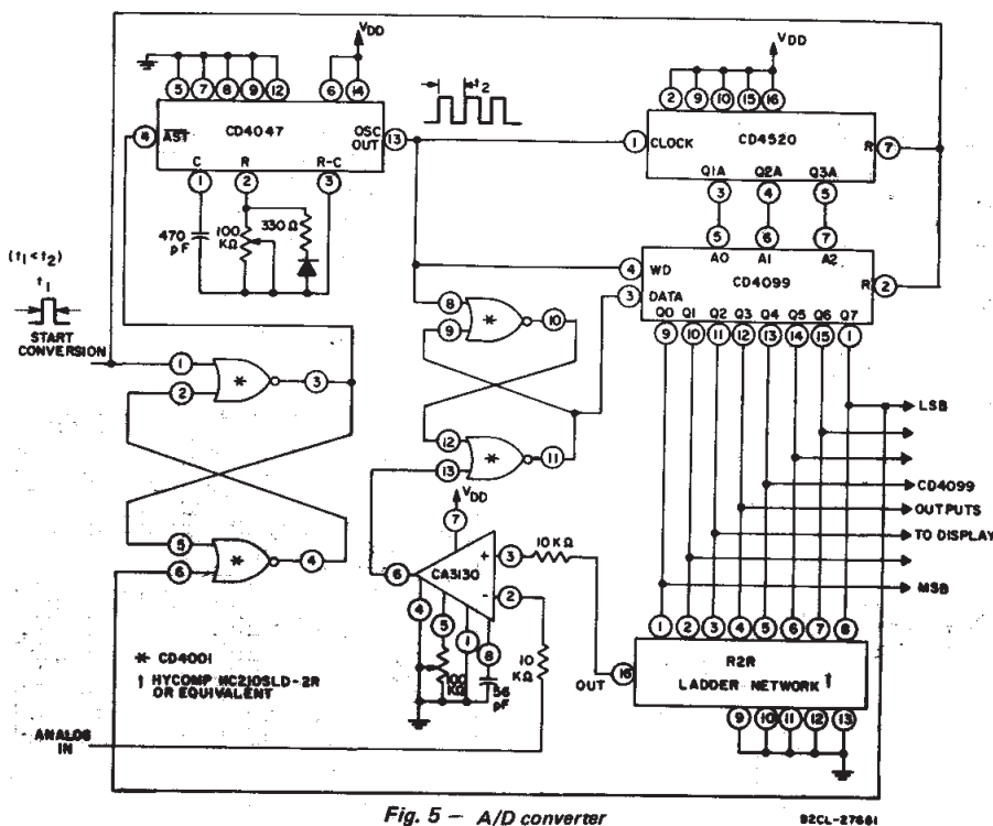
Fig. 5 — A/D converter
