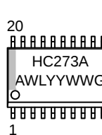
SOIC-20
