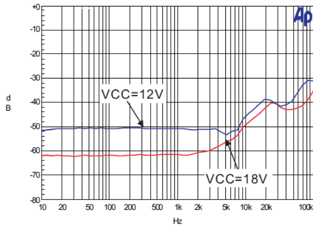
7. PSRR
