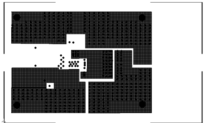
Figure 12. SP7655EB PC Layout 3 rd Layer
