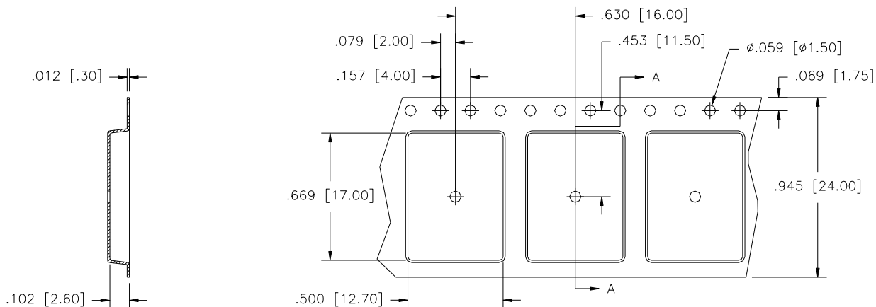
SECTION A-A
