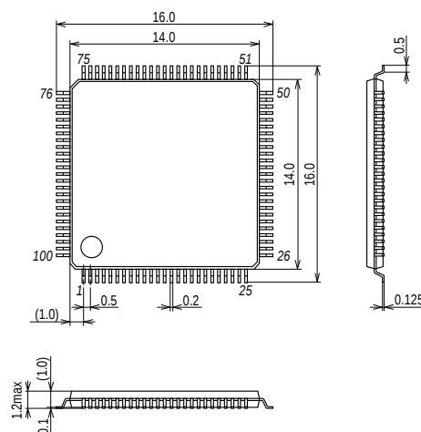
TQFP100(14X14)
