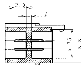
SECT A-A
