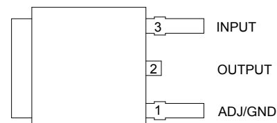
TO252-2 (5)
