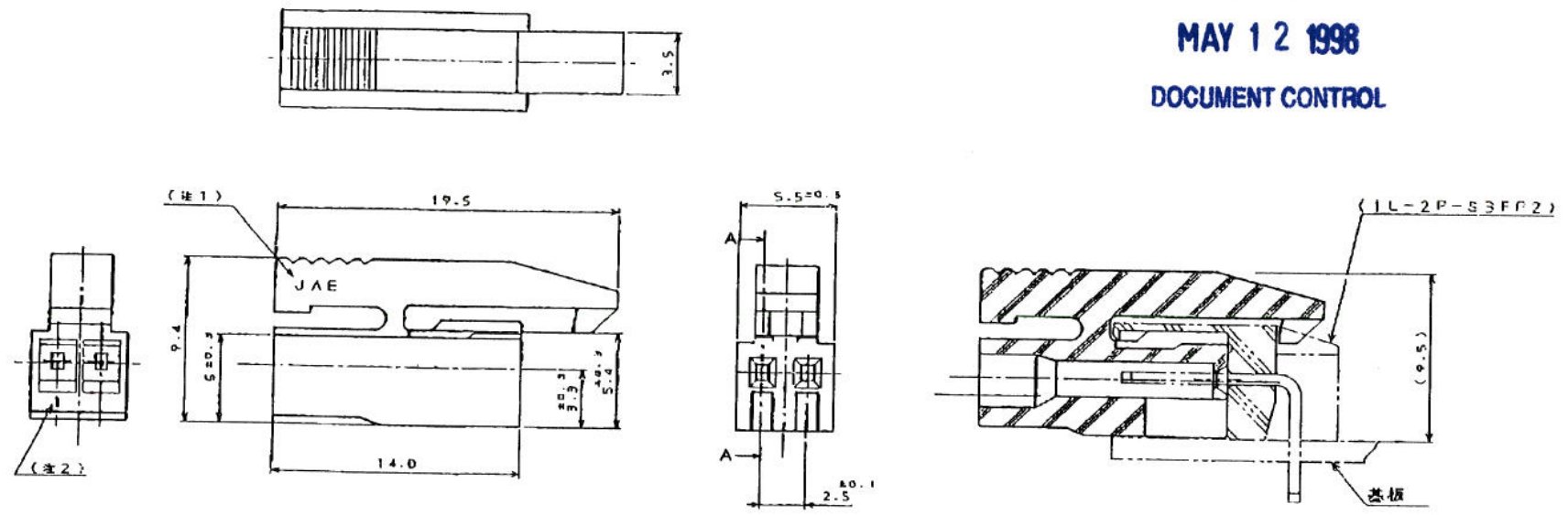
断面A-A及び組合せ状態図
