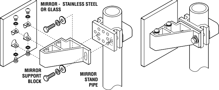
MIR45-BKT
