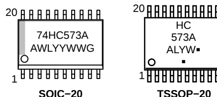
SOIC-20
