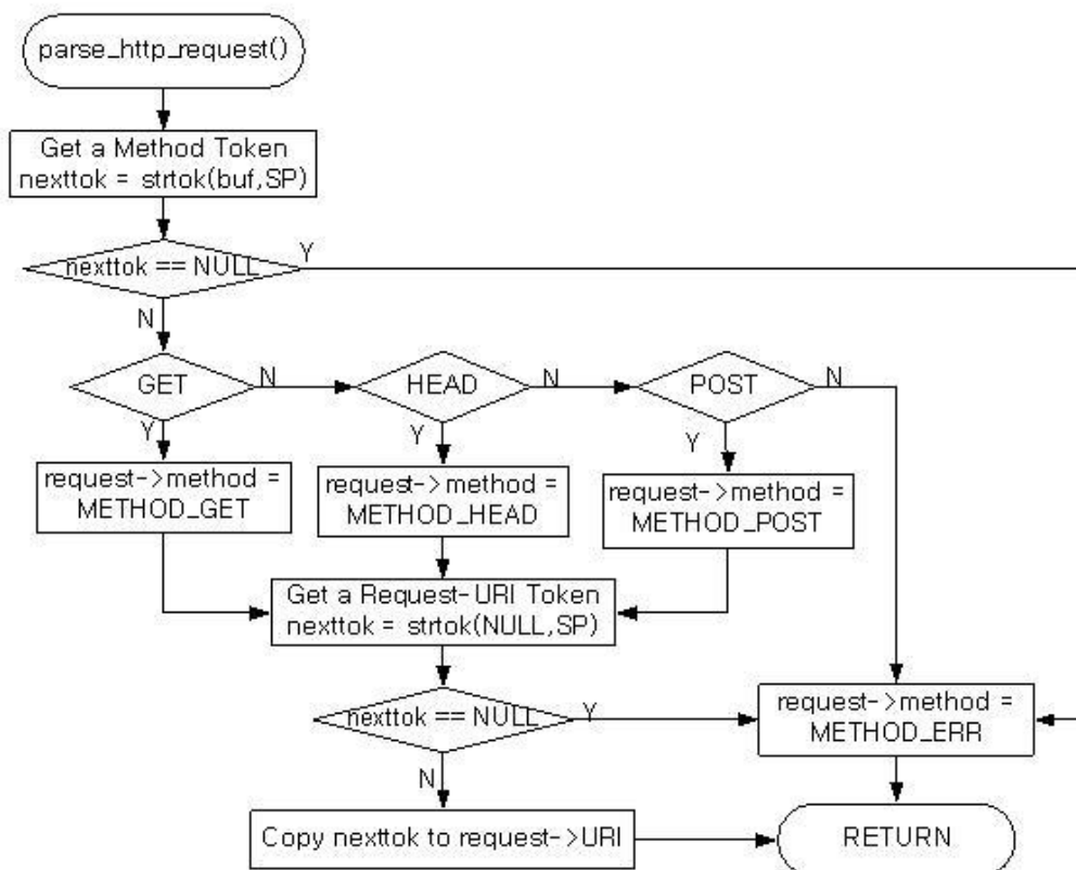
<Fig 3.20: parse_http_request() >
