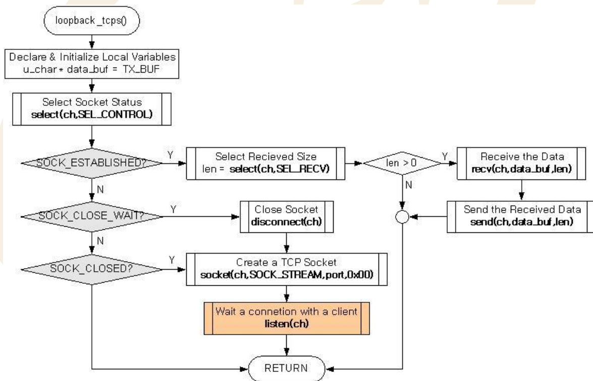
< Fig 3.14 : loopback_tcps() >
