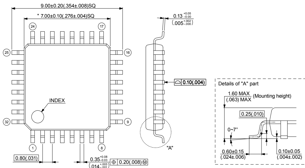
32-pin plastic LQFP (FPT-32P-M30)
