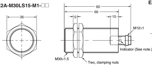
E2A-M30LS15-M1-□□
