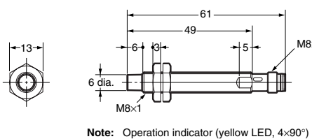
E2A-S08LN04-M5-□□
