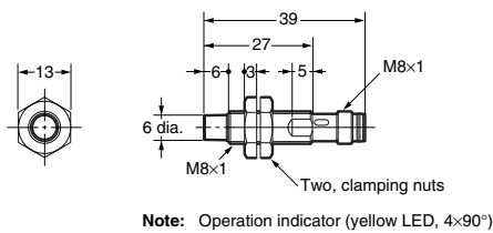
E2A-S08LN04-M5-□□
