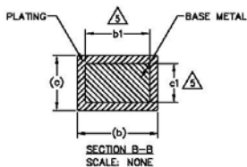
SECTION B-E SCALE: NONE
