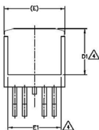
VIEW A-A
