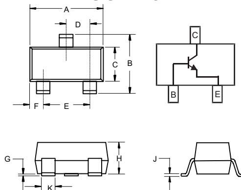
DIMENSIONS
