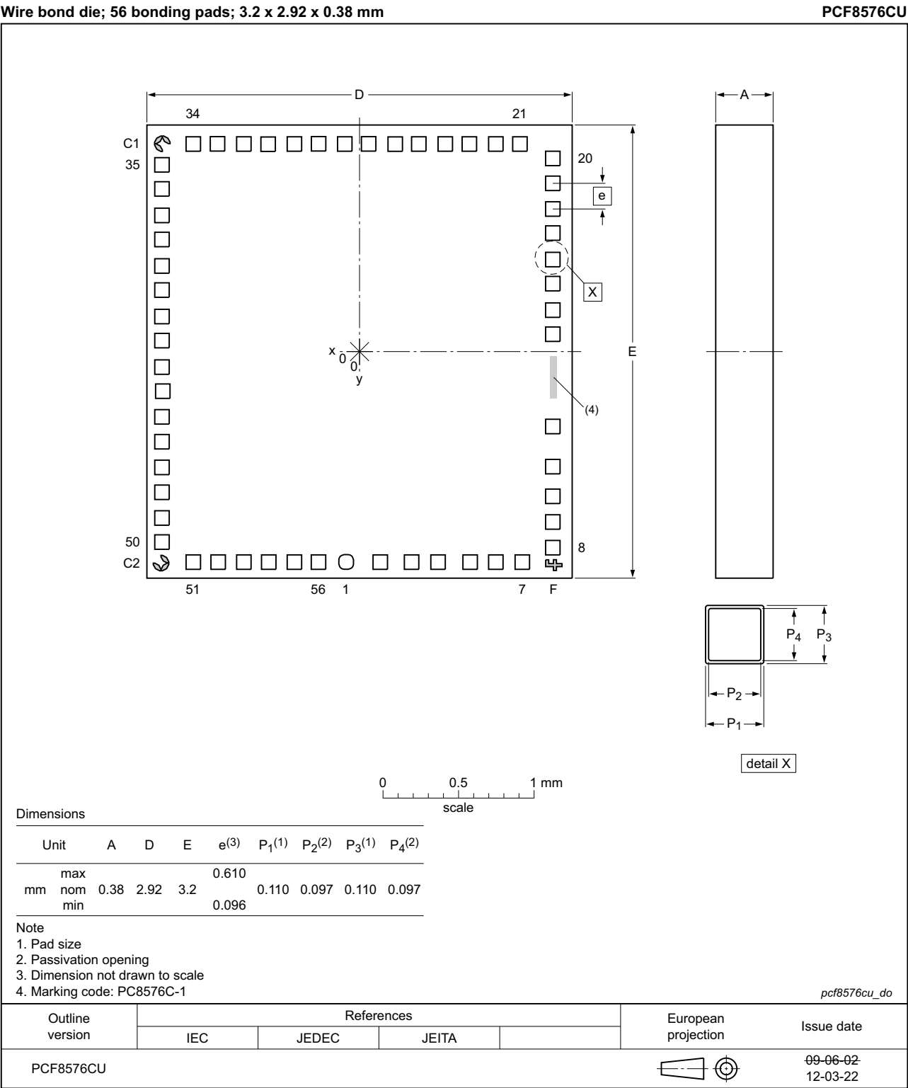
Fig 36. Bare die outline of PCF8576CU/F1
