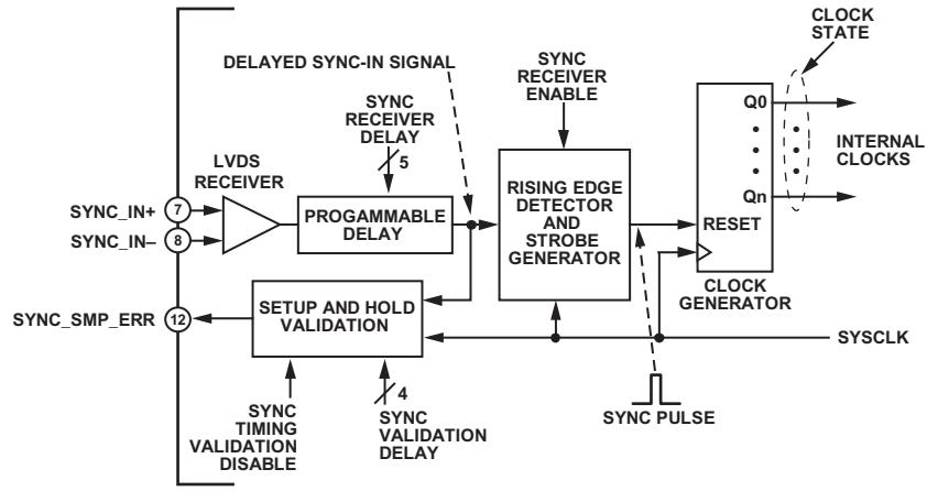
图52. 同步接收器框图
