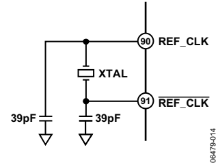
图31. 晶体连接图
