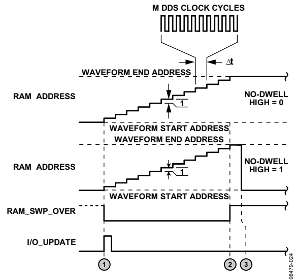
图43. 上斜坡时序图
