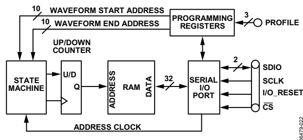
图41. RAM数据加载/读取操作
