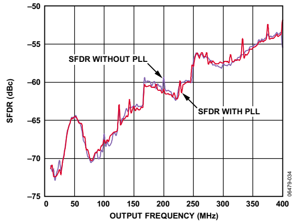
图6. 宽带SFDR与输出频率的关系 (PLL参考时钟频率 = 15.625 MHz 64 )
