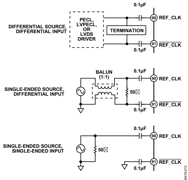
图32. 直接连接图
