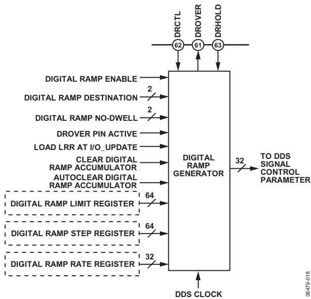
图37. 数字斜坡功能框图
