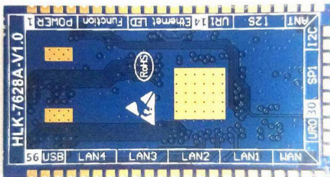
HLK-7628A 背面图
