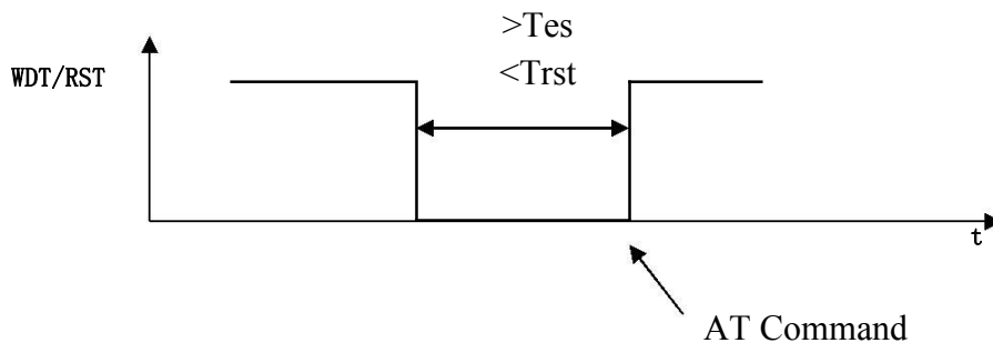
图 8. WDT/RST 退出透传模式
