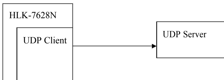
图 13.UDP Client
