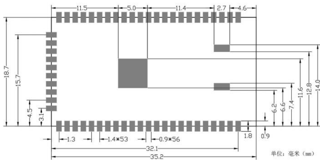
建议封装尺寸图
