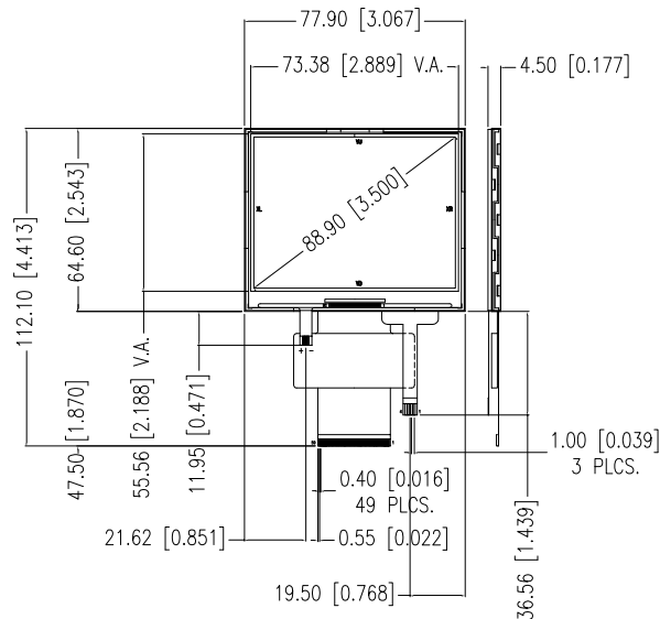
3.5" Module - LCT-H320240M35WT
