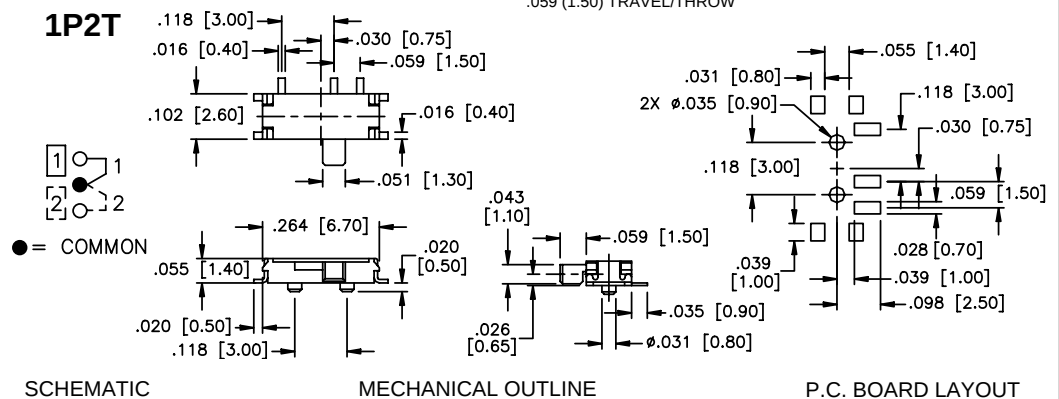
RIGHT ANGLE ACTUATOR
