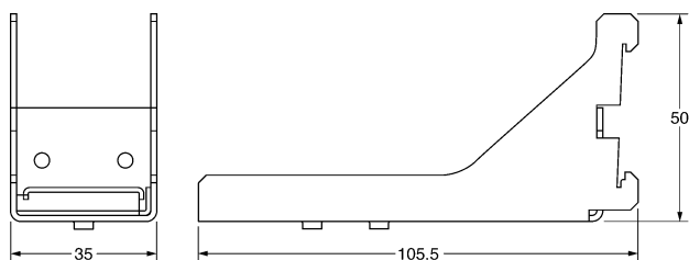
SRT2-ATT01
