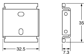
SRT2-ATT02
