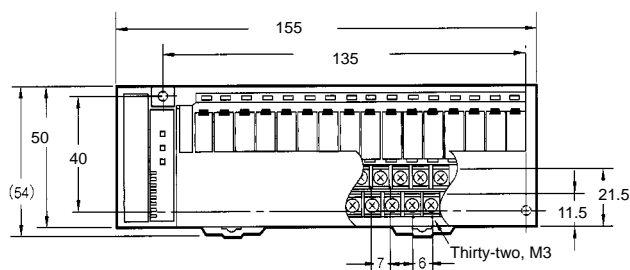
Two, 4.2 dia. or M4 41 \pm 0.2 135 \pm 0.2
