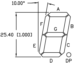
DIGIT DETAIL
