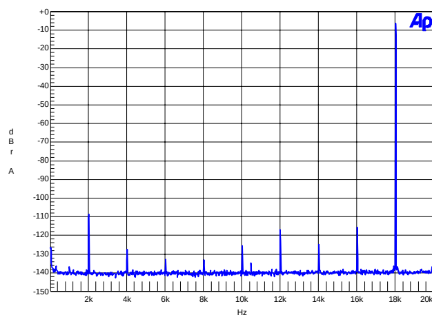
Figure 20. FFT (IMD 96 kHz)
