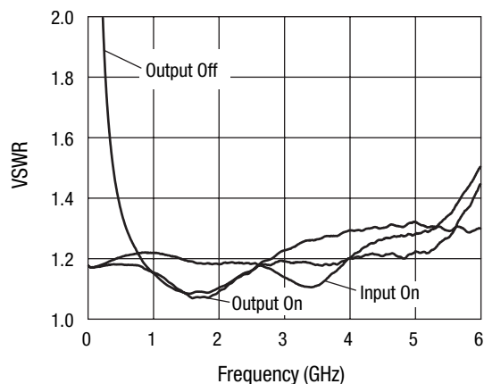
VSWR, 25 °C
