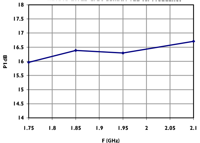
P1dB
