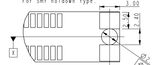
DETAIL E SCALE 3.000
