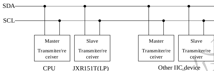
图 11-3 IIC 系统配置
