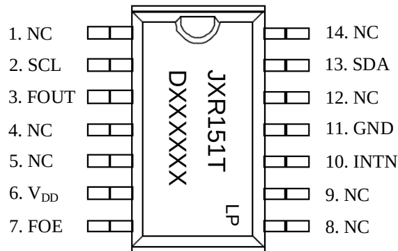
图 4-1 JXR151T(LP)封装形式
