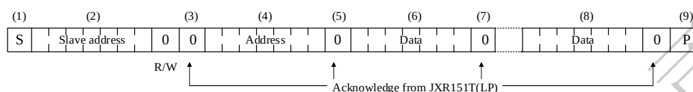
图 11-4 指定地址写操作
