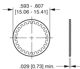
LOCKWASHER
