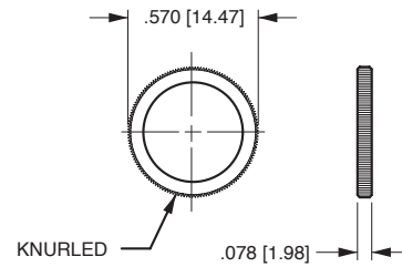
STANDARD FACENUT
