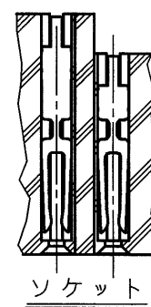
断面A-A (尺度 2/1)
