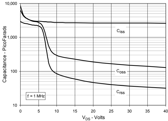
Fig. 13. Capacitance
