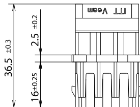
Receptacle, 6 poles
