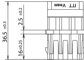
Receptacle, 3 poles
