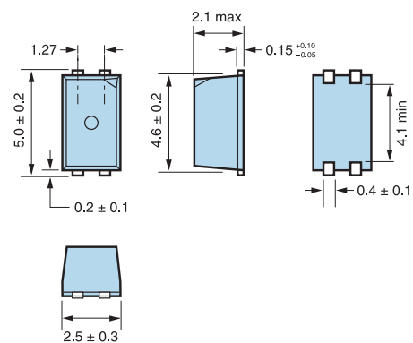
4-Pin Mini Flat
