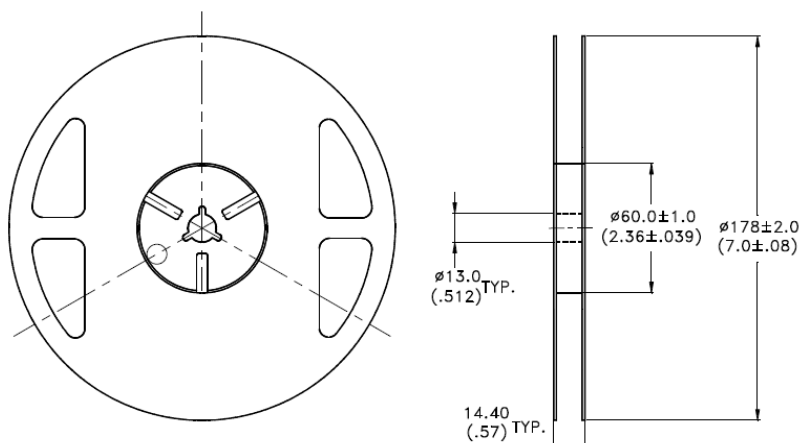
Reel dimensions Unit:mm
